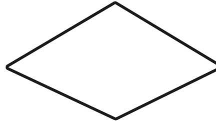
rhombus
