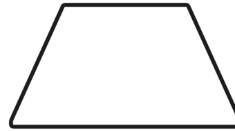
trapezium
